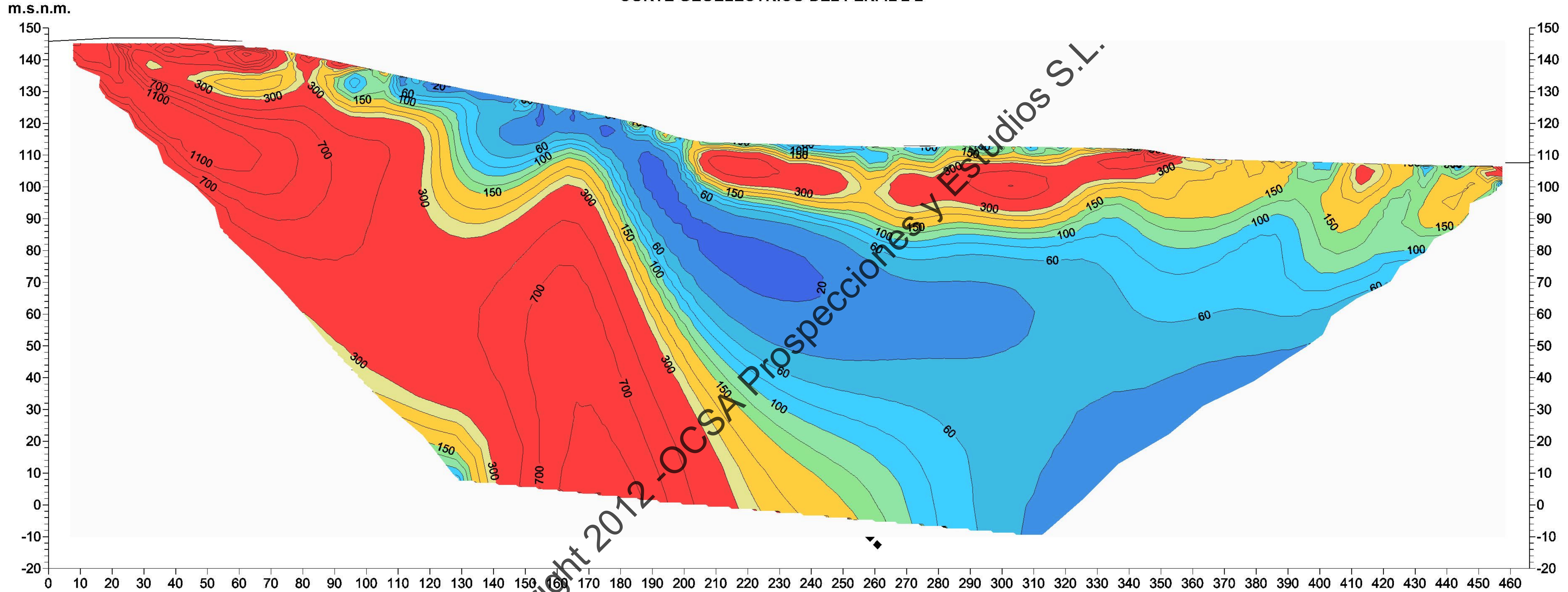
CORTE GEOELÉCTRICO DEL PERFIL 2-2
